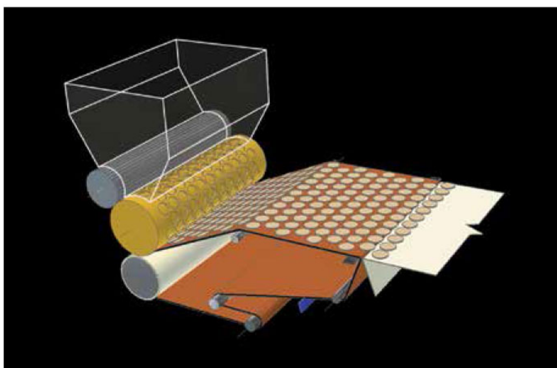
Diagrama de un moldeador rotatorio
